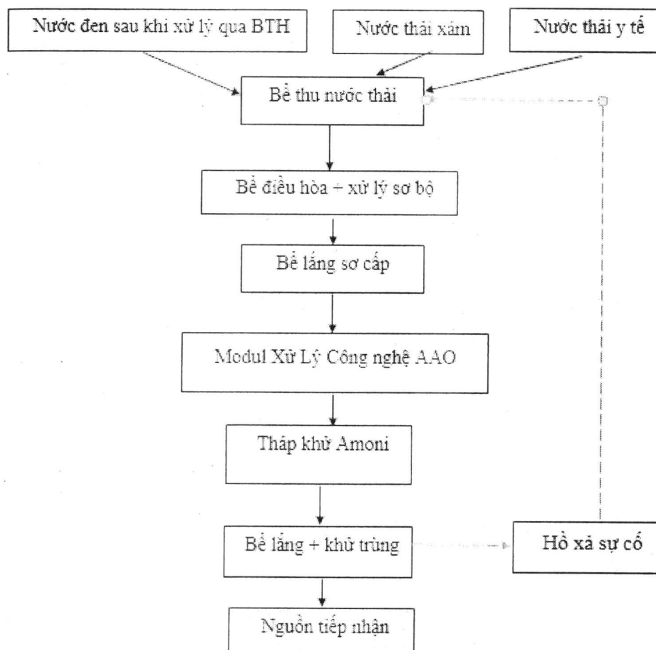
Hình: Sơ đồ công nghệ HTXLNT của Bệnh viện ĐKKV Bắc Quảng Bình
