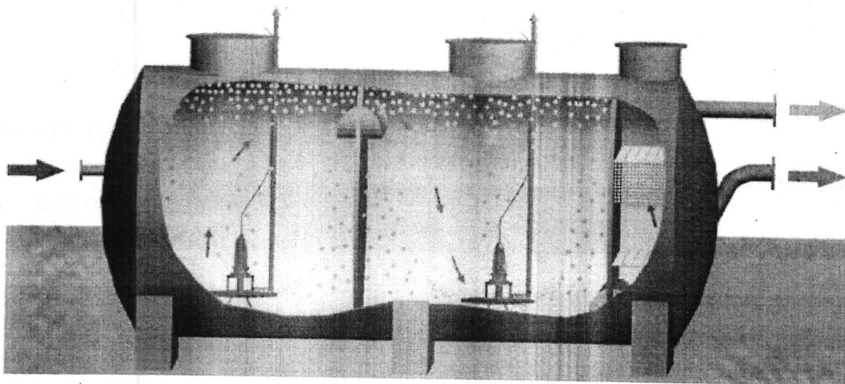
Hình: Hệ thống xử lý chất thải lỏng y tế - Loại Hợp khối
